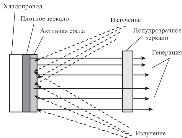
Рис.6. Излучающее зеркало Басова (дисковый лазер).
